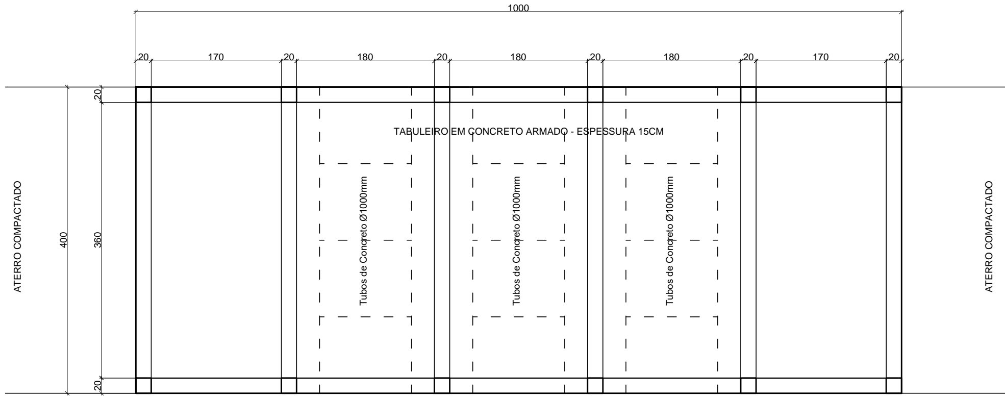
PLANTA BAIXA ESC. 1:50
