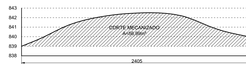
PERFIL TRANSVERSAL ESC. 1:200
